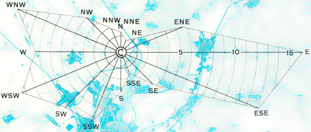
Windhäufigkeit in %
