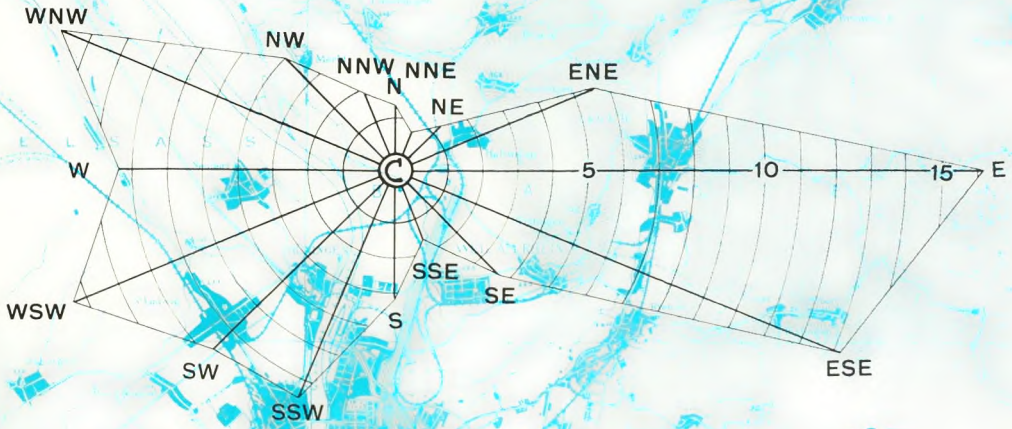
Windhäufigkeit in %
